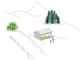
Gruppen- Weidehaltung 4.6%
