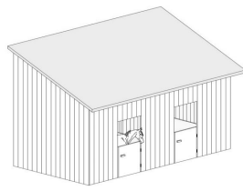
Aussenbox 8.7%
