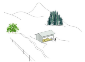
Weidehaltung 7.1%
