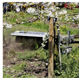
Mechanische Baumstreifenpflege (von links nach rechts: Hackgerät [«Ladurner»], Rollhacke, Fadengerät, Bürstengerät [Foto Bürstengerät: A. Buser, LZ Ebenrain]).
