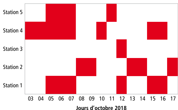
Figure 4 | Périodes de forte concentration de particules de la taille des spores de Plasmopara viticola (sphéroïdes de 16 à 20 µm), sur les cinq stations de mesure de Dardagny (GE) (fig. 1).
