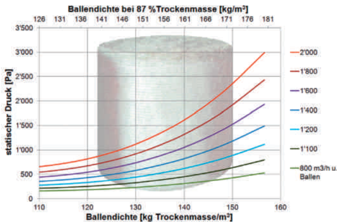
Abb. 16: Erforderlicher Druck für 1,5m Ballendurchmesser bei Wiesenheu.
