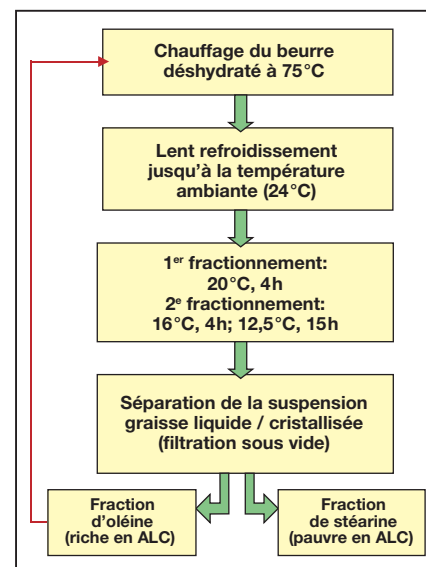
Fig. 3. Schéma du procédé de fractionnement.
