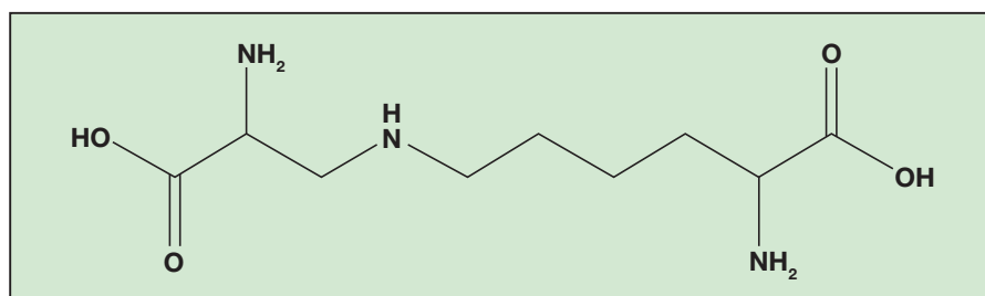
Fig. 1. Formule chimique de la lysinoalanine.
