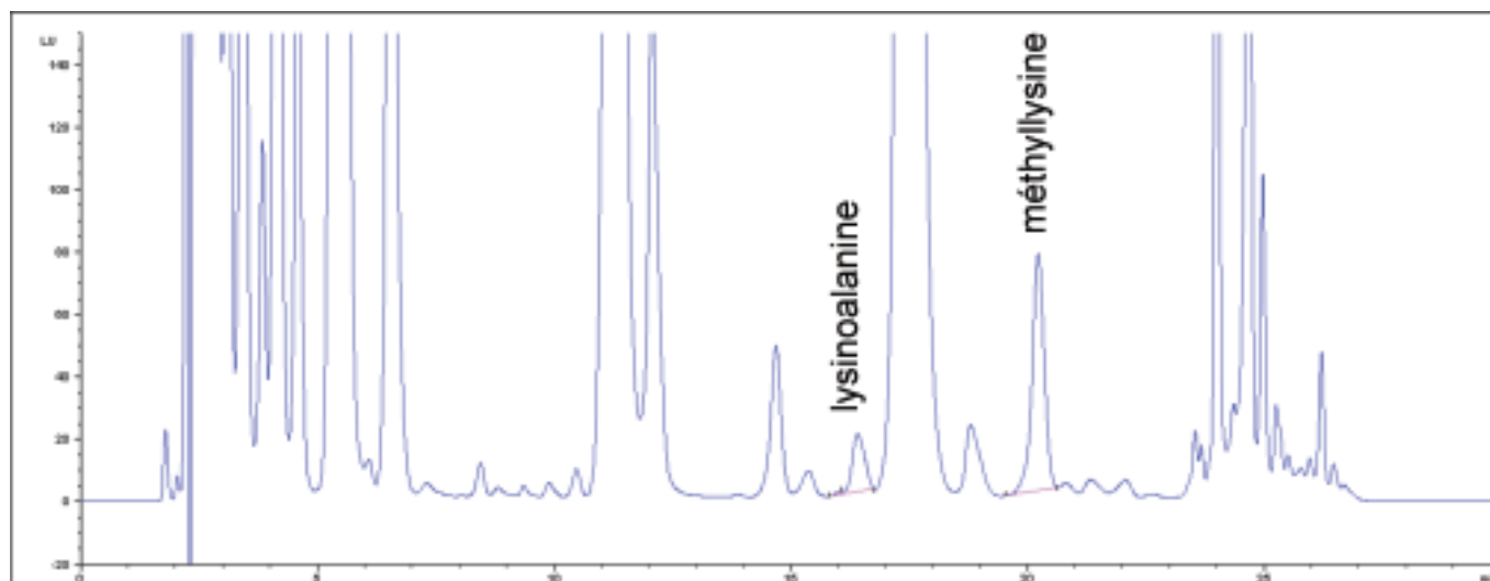
Fig. 2. Séparation par HPLC d'un échantillon de poudre de lait entier contenant de la lysinoalanine ajoutée et de la méthyllysine comme standard interne.
