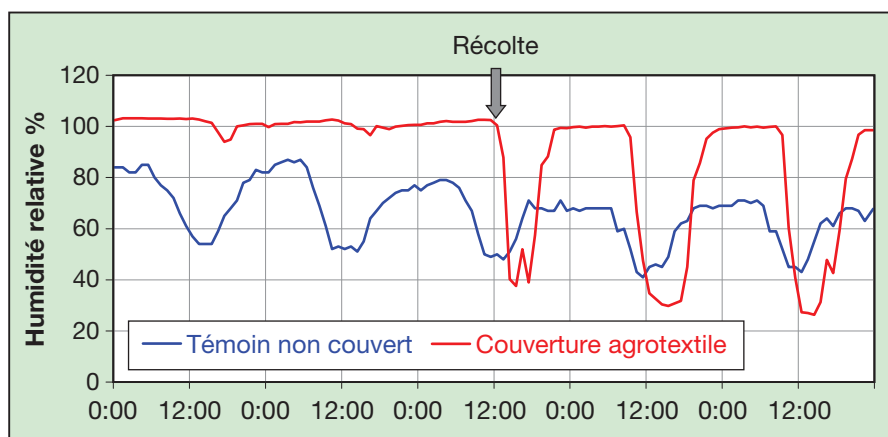
Fig. 6. Courbes d'humidité relative avec agrotextile (en rouge) et sans agrotextile (en bleu) enregistrées dans une culture de melisse à Brunson du 31 août au 4 septembre en 2004; la récolte a eu lieu le 2 à 13 heures.
