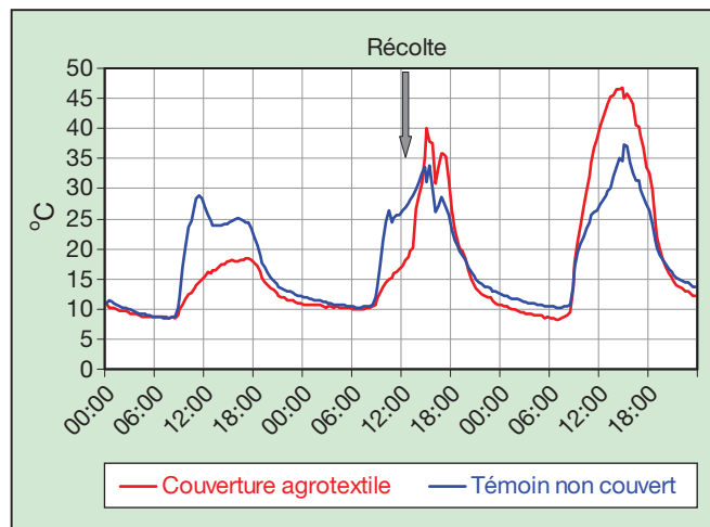
Fig. 5. Courbes de températures avec agrotextile (en rouge) et sans agrotextile (en bleu) enregistrées dans une culture de melisse à Brunson du 1 er au 3 septembre en 2004; la récolte a eu lieu le 2 à 13 heures.
