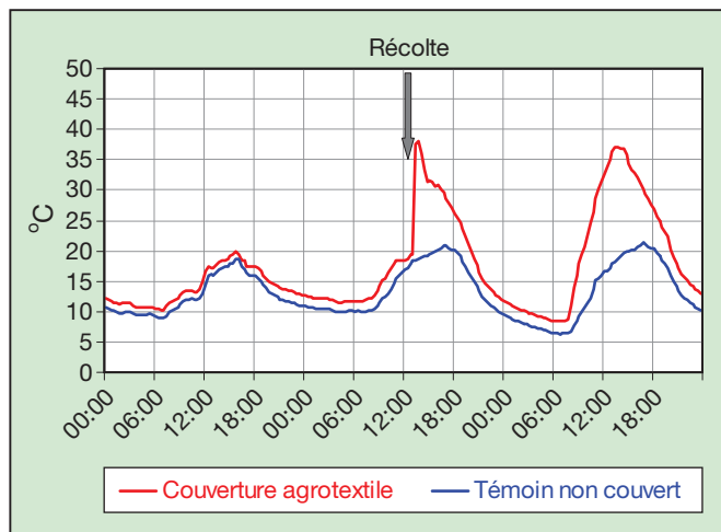
Fig. 4. Courbes de températures avec agrotextile (en rouge) et sans agrotextile (en bleu) enregistrées dans une culture de melisse à Brunson du 27 au 29 mai en 2004; la récolte a eu lieu le 28 à 13 heures.
